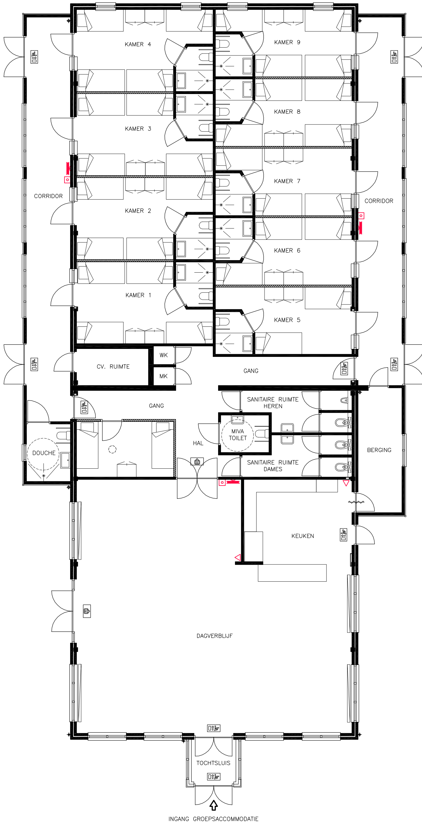
PLATTEGROND GROEPSACCOMMODATIE "DE LANDERIJ"
